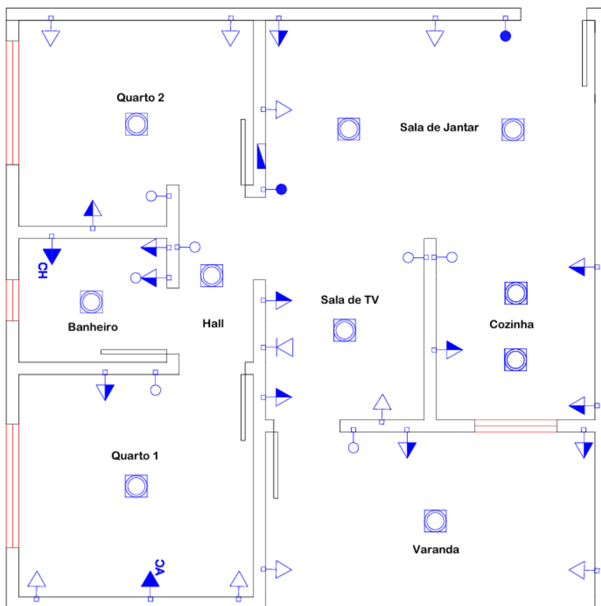
Figura 5 - Representação dos pontos de tomada e iluminação
