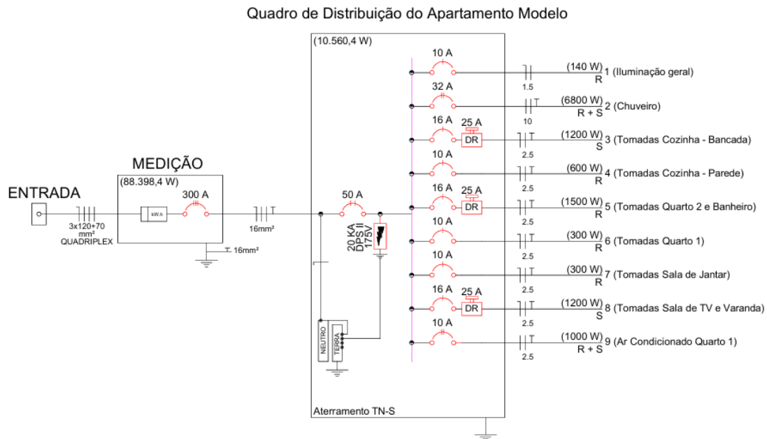
Figura 7 - Diagrama unifilar do apartamento modelo
